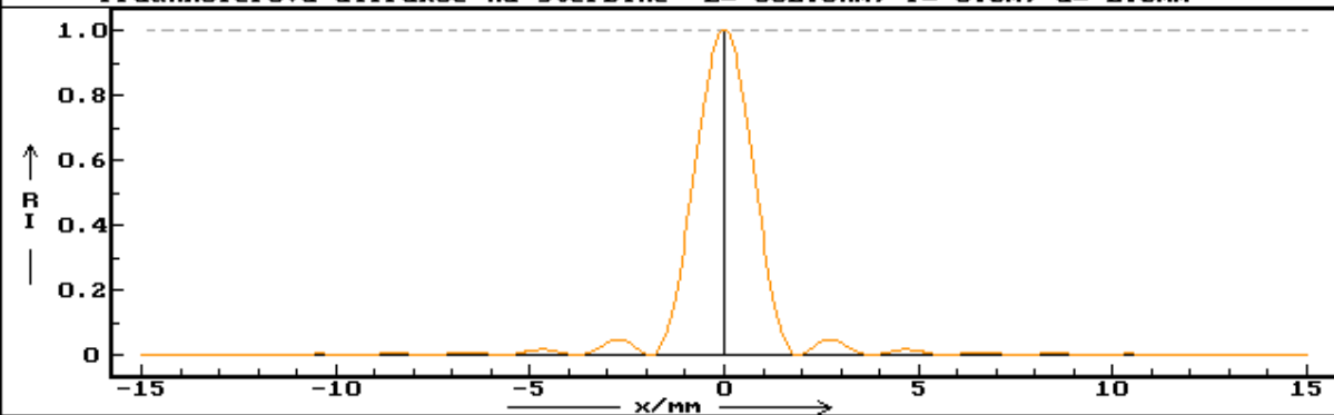
Fraunhoferova difrakce na štěrbině L = 632.8\text{nm} , f = 6.0\text{m} , a = 2.0\text{mm}
