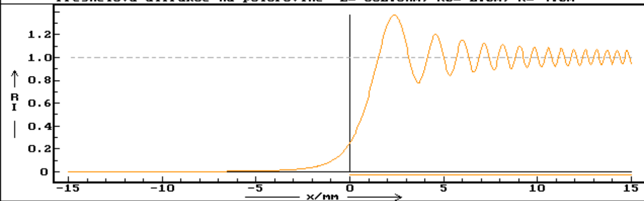
Fresnelova difrakce na polorovině L = 632.8\text{nm} , R_0 = 2.0\text{m} , R = 4.0\text{m}
