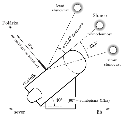
Obr. 2 — Pohled na budík od západu ve 12 h PMSČ, když je Slunce přesně na jihu. Výška Slunce nad rovníkem (deklinace) je největší při letním slunovratu (+23,5°), nejmenší při zimním slunovratu (-23,5°), při jarní a podzimní rovnodennosti je nulová. Číselník je vzhledem k vodorovné rovině skloněn stejně jako rovník o úhel (90^\circ - \text{zeměpisná šířka stanoviště}) , tj. přibližně 40°.
