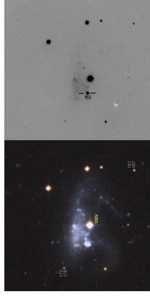
Obr. 1 — Vlevo snímek hostitelské galaxie NGC 3239 bez supernovy; není-li uvedeno jinak, byly snímky převzaty z [3]. Vpravo se supernovou SN 2012A v době objevu 7. 1. © Tim Puckett; převzato z ( http://www.possdata.com/PSNJ10250739+1709146.jpg ).
