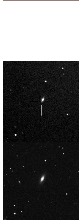
Obr. 8 — Vlevo snímek hostitelské galaxie NGC 5611 bez supernovy. Vpravo pak se supernovou SN 2012ei brzy po objevu, 23. 8. © Yoji Hirose; převzato z ( http://www.flickr.com/photos/sn-images/7848018228/ ).
