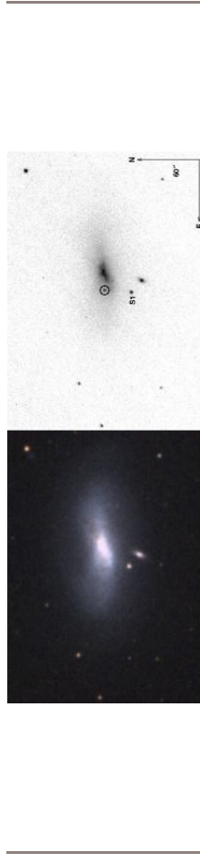
Obr. 6 — Vlevo snímek hostitelské galaxie NGC 4424 bez supernovy. Vpravo se supernovou SN 2012cg v době objevu 17. 5. © LOSS; převzato z ( http://astro.berkeley.edu/~cenko/public/finders/NGC4424.gif ).
