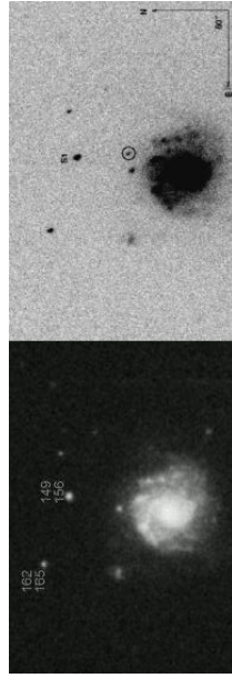
Obr. 2 — Vlevo snímek hostitelské galaxie NGC 1309 bez supernovy. Vpravo se supernovou SN 2012Z v době objevu 29. 1. © LOSS; převzato z ( http://astro.berkeley.edu/bait/public_html/2012/sn2012Z.html ).
