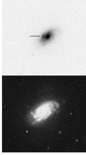
Obr. 7 — Vlevo snímek hostitelské galaxie NGC 1084 bez supernovy. Vpravo se supernovou SN 2012ec v den objevu 11. 8. © Berto Monard; převzato z ( http://www.rochesterastro-my.org/sn2012/n1084s1.jppe ).
