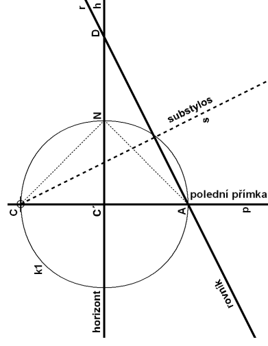
Obr. 14 — Konstrukce horizontu a rovníku.
