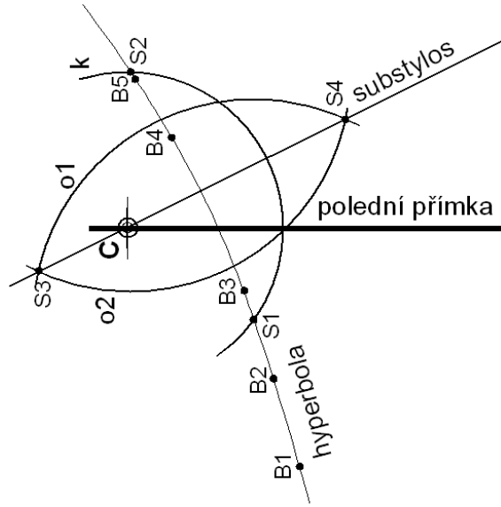
Obr. 13 — Určení směru substylu.
