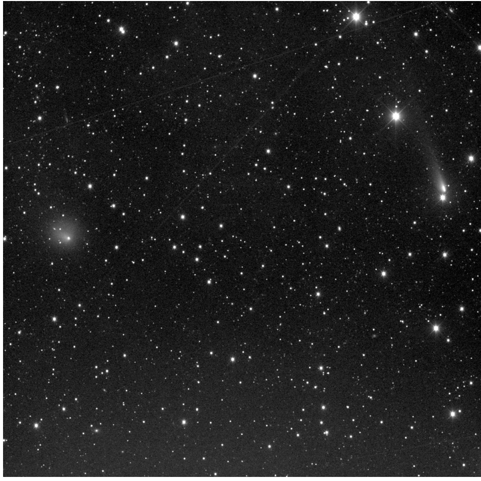
Obr. 4 — Ve spodní části snímku se nachází kometa 81P/Wild 2, je protažená s výrazným chvostem. Naproti, u horního okraje, je kometa 29P/Schwassmann-Wachmann 1, více kruhového vzhledu. Nedaleko od ní, napravo těsně u stopy družice, je patrná slabá protáhla skvrnka, kometa C/2009 U6 (LINEAR). Snímek pořízený 27,18 října 2009 UT je kompozicí devíti 120 s expozic. Převzato z ( http://astrosurf.com/obsdauban/pages/PO9U6.html ).
