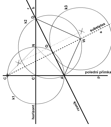
Obr. 15 — Sklopení roviny rovníku do roviny stěny.
