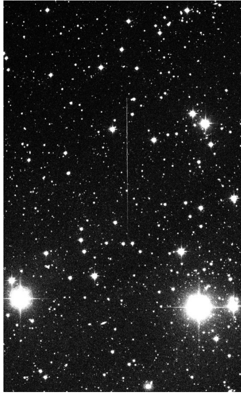
Obr. 2 — Pohyb planetky 2008 TC 3 od 1 h 45 min 23 s UTC až do zmižení ve stínu planety Země v 1 h 47 min 30 s UTC. Planetka byla v čase expozice vzdálena 29 600 km a pohybovala se rychlostí 7,61 km/s. Proměnná jasnost stopy planetky byla zapříčiněna její rotací. © La Sagra Sky Survey.
