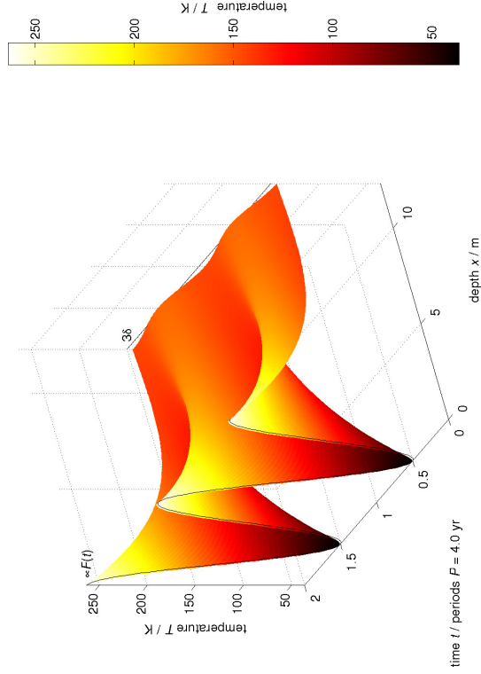
Obr. 12 — Třizměrný náčrt závislosti hloubky x , času t a teploty T , jak vyplývá z jednorozměrného modelu (13). Vlastnosti materiálu odpovídají bazaltické hornině (viz tab. 2), s tepelnou vodivostí K = 1 \text{ W}/(\text{m}\cdot\text{K}) . Amplituda \mathcal{E}_1 zářivého toku je polovinou rovnovážného toku \mathcal{E}_0 na 2,5 AU od Slunce; frekvence f toku \mathcal{E}(t) odpovídá orbitální periodě P = 4 \text{ y} . Tok je kreslen jako tenká linka v rovině (t, T) a je škálováný stejně jako amplituda T_1(0) povrchové teploty. Tepelné zpoždění mezi dopadajícím tokem \mathcal{E}(t) a povrchovou teplotou T(0, t) je zřetelné ( \phi_{\text{th}} \approx -4^\circ ).
