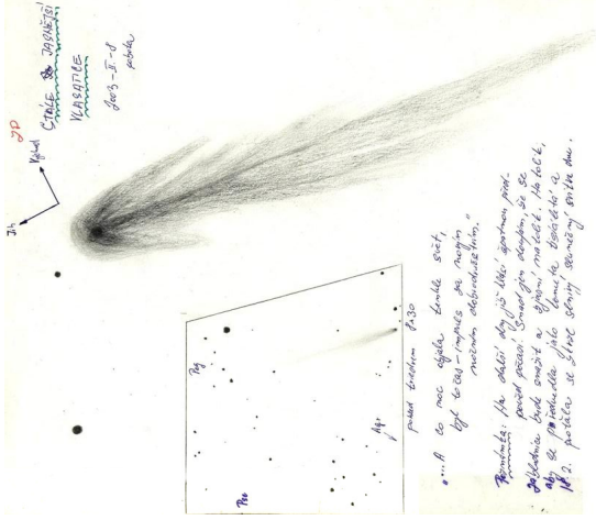
Obr. 7 — Komete C/2002 V1 NEAT se rychle stávala vlasatící.
