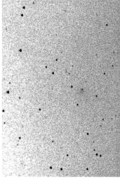
Obr. 3 — Snímek komety 205P/Giacobini pořízený 11. 9. 2008 v 18 h 40 m UT pomocí 0,40 m dalekohledu JST, CCD ST-7 s filtrem R na královhradecké hvězdárně. Jedná se o kompozici astrometrických snímků 2 × 30 s. Měsíční svit způsobil nerovnoměrné pozadí snímku, přesto je kometa pěkně viditelná — jak silně až stelární centrální zhuštění, i velmi slabý difúzní závoj rozkládající se východním směrem.
