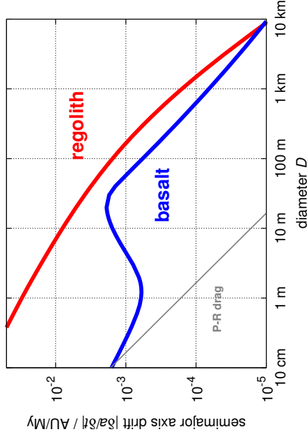
Obr. 16 — Suma absolutních hodnot |da/dt| denního a ročního driftního velké poloosy v závislosti na velikosti, vypočtená pro kulová tělesa, střední hodnotu šikmosti \gamma = 135^\circ a dva různé materiály z tab. 2: bazalt a regolit, tzn. materiál s vysokou a nízkou tepelnou vodivostí. Neočekáváme, že by existovala příliš malá tělesa pokrytá regolitem, proto změny velké poloosy větší než 10^{-2} AU/My zřejmě nejsou realistické. Drift způsobený Poyntingovým–Robertsonovým jevem je také zakreslen; převažuje pro velikosti menší než 10 cm.
