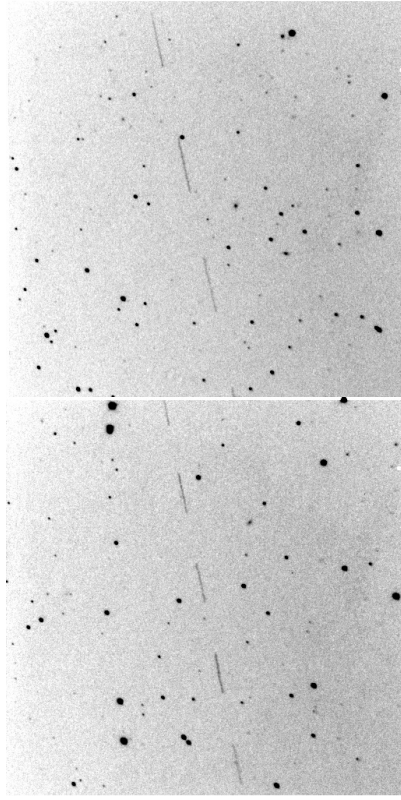
Obr. 1 — Planetka 2008 TC 3 v 1 h 32 min a 1 h 42 min UTC. Na expozicích trvajících 10 s je planetka značně protažená. Během 10 minut, které uplynuly mezi dvěma snímky je evidentní zrychlení pohybu způsobené gravitací Země. © Eric Allen, Observatoire du Cégep de Trois-Rivières.
