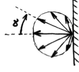
Obr. 13 — Lambertův zákon rozptylu, znázorněný jako rozptylový diagram ve tvaru koule přiléhající k povrchu.
