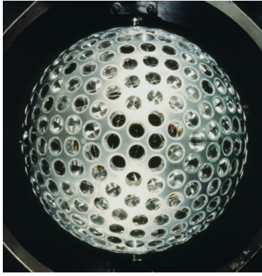
Obr. 9 — Geodynamická družice LAGEOS — koule s poloměrem 30 cm a hmotností 410 kg, pokrytá 426 retro-reflektory, které umožňují její sledování lasery z pozemských observatoří. Obíhá ve výšce 5 900 km nad Zemí. Viz též tab. 1. Převzato z [1].
