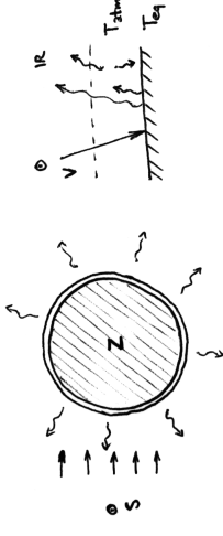
Obr. 10 — Zeměkoule s tenkou atmosférou.
