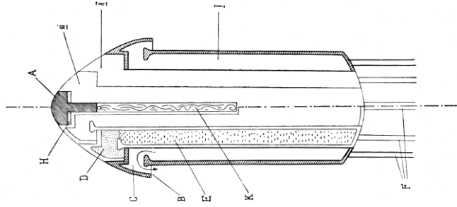
Obr. 9 — Výšková raketa.
