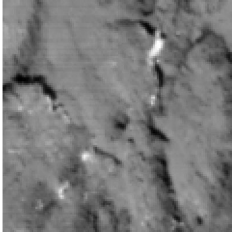
Obr. 2 — Jádro 30 s před dopadem.
