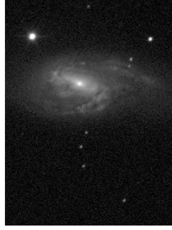
Obr. 8 — M 66 v noci 23. 11. 1998. Sledována CCD kamerou PixCel 255 (ST-5C) a dalekohledem Newton 250 mm (f/5) se zorným polem 9' \times 7' . Foto Miroslav Brož.
