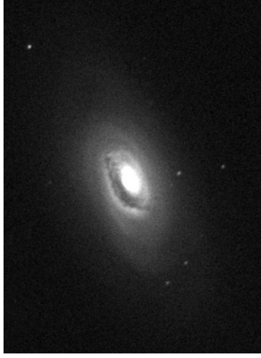
Obr. 10 — Galaxie M 64 zachycená 180s expozicí v noci 24. 12. 1998 ve 3 h 1 min UT. Foto Miroslav Brož.
