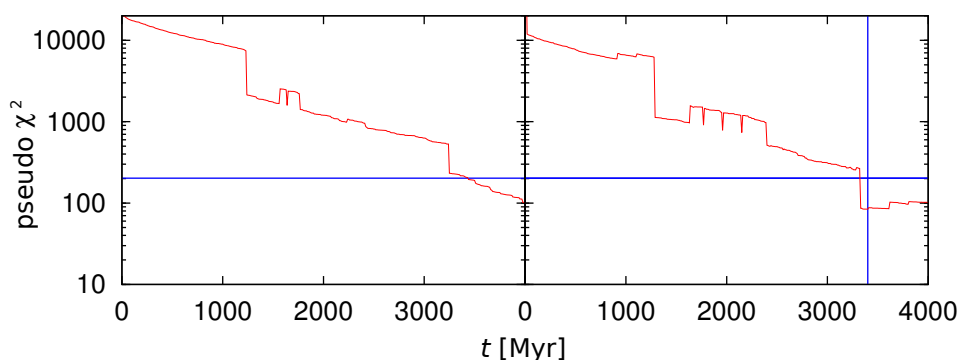
Obrázek 4.6: Časový vývoj (pseudo- \chi^2 ) pro rodinu Fringilla. Vertikální modré čáry označují čas, kdy je \chi^2 nejmenší; horizontální čáry označují dvojnásobek minimální hodnoty \chi^2 . Na levém obrázku je vyznačena situace pro rychlost srážky 3 km/s, úhel 45° a rozměr mateřského tělesa 120 km. V tomto případě se rozdělení nejlépe shodují v konečném čase, tedy t = 4 Gyr. Pod hladinou dvojnásobku minimální hodnoty \chi^2 je to t > 3,43 Gyr. Na pravém panelu je rychlost srážky 5 km/s, úhel 15° a rozměr mateřského tělesa 135 km. Zde se rozdělení nejlépe shodují v t = 3,40 Gyr a pod hladinou dvojnásobku minimální hodnoty \chi^2 je t > 3,33 Gyr.
