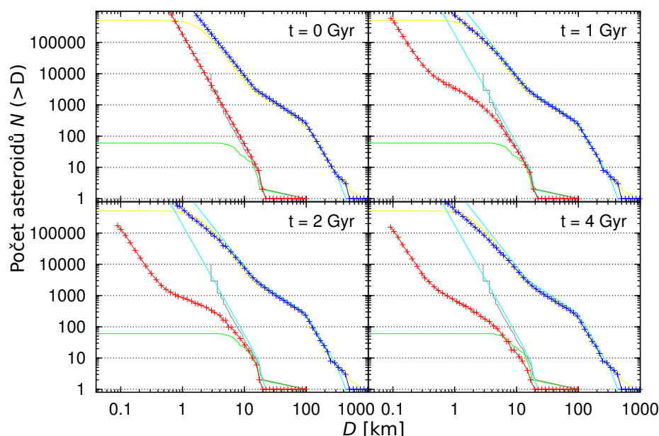
Obrázek 4.5: Kolizní vývoj kumulativního rozdělení velikostí těles rodiny Fringilla modelovaný programem Boulder. Popis viz obrázek 4.10. V tomto případě se jedná o rychlost srážky 5 km/s, úhel 15° a rozměr mateřského tělesa 135 km. Na obrázcích je znázorněna situace na počátku vývoje, po 1 Gyr, po 2 Gyr a po 4 Gyr.
