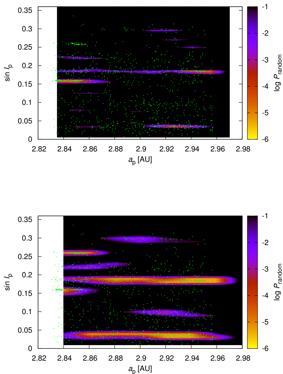
Obrázek 1.4: Barevné znázornění statistické významnosti shluků těles. Na diagramu vlastní velká polosa a_p a vlastní sklon \sin i_p jsou body vyznačena tělesa v rozsahu vlastních excentricit e_p = 0,10 až 0,12 . Barevná škála ukazuje pravděpodobnost, že je shluk v daném místě náhodný. První obrázek je sestaven pro velikost boxu a_p : e_p : i_p rovnou 0,03 \text{ AU} : 0,01 : 0,01^\circ a 100 000 pokusů. Druhý obrázek znázorňuje výsledek pro velikost 0,04 \text{ AU} : 0,02 : 0,02^\circ a 200 000 pokusů. Jedná se tedy o stejné nastavení jako v případě obrázku 1.2.
