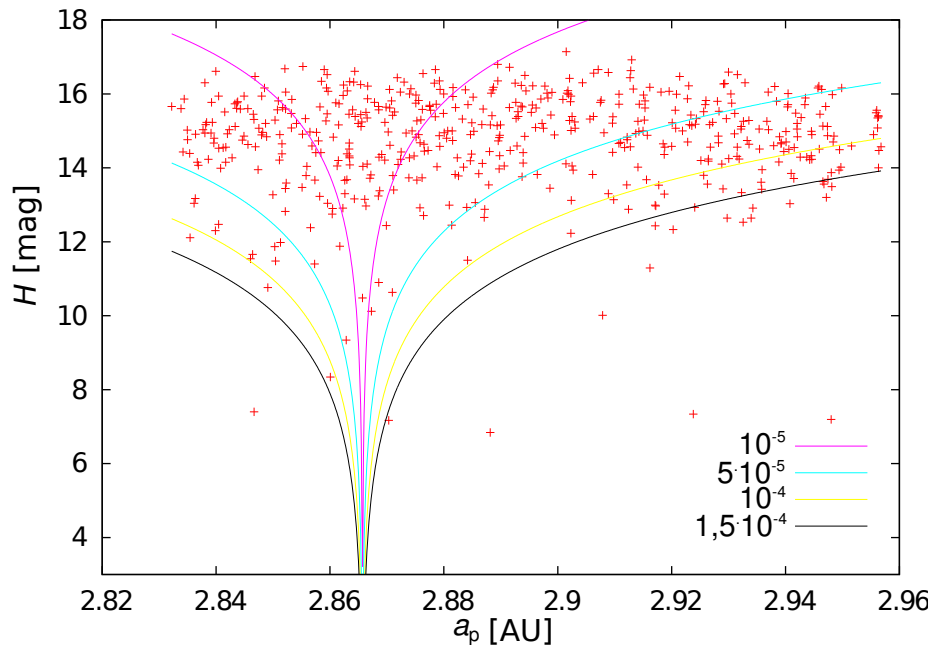
Obrázek 3.3: Ukázka použití metody aH pro vyřazování pravděpodobně přimísených těles. Červenými křížky jsou vyznačeny polohy těles v diagramu vlastní velká poloosa a versus absolutní magnituda H . Barevné linie odpovídají rovnici 3.5. V pravém dolním rohu jsou hodnoty parametru C . Tělesům, která nejsou členy rodiny, by příslušelo příliš velké C , výrazně vyšší, než shluk ostatních.
