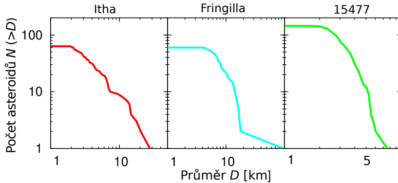
Obrázek 2.8: Pozorovaná kumulativní rozdělení velikosti vybraných rodin Itha, Fringilla a 15477. Rozměry těles byly vypočteny z průměrného albeda členů rodiny a jejich absolutní hvězdné velikosti.
