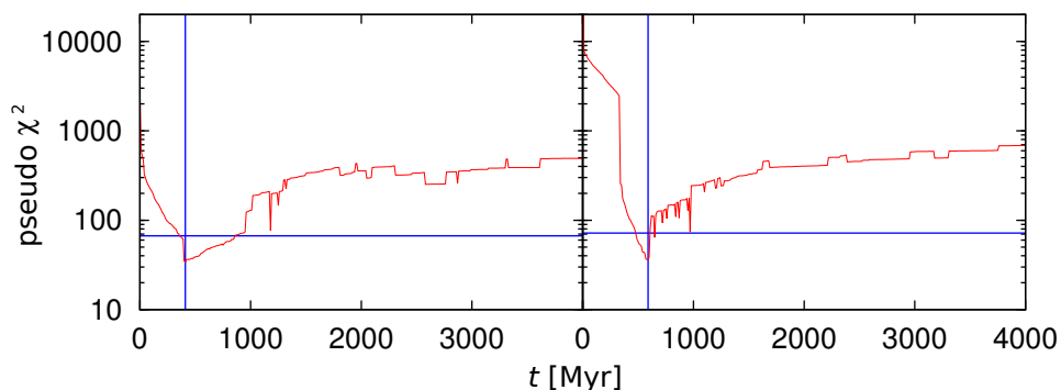
Obrázek 4.9: Časový vývoj (pseudo- \chi^2 ) pro rodinu 15477. Vertikální modré čáry označují čas, kdy je \chi^2 nejmenší; horizontální čáry označují dvojnásobek minimální hodnoty \chi^2 . Na levém obrázku je vyznačena situace pro rychlost srážky 4 km/s, úhel 45^\circ a rozměr mateřského tělesa 40 km. V tomto případě se rozdělení nejlépe shodují v čase t = 0,41 Gyr. Pod hladinou dvojnásobku minimální hodnoty \chi^2 je to t \in [0,35; 0,86] Gyr. Na pravém panelu je rychlost srážky 7 km/s, úhel 30^\circ a rozměr mateřského tělesa 70 km. Zde se rozdělení nejlépe shodují v t = 0,59 Gyr a pod hladinou dvojnásobku minimální hodnoty \chi^2 je t \in [0,47; 0,61] Gyr.
