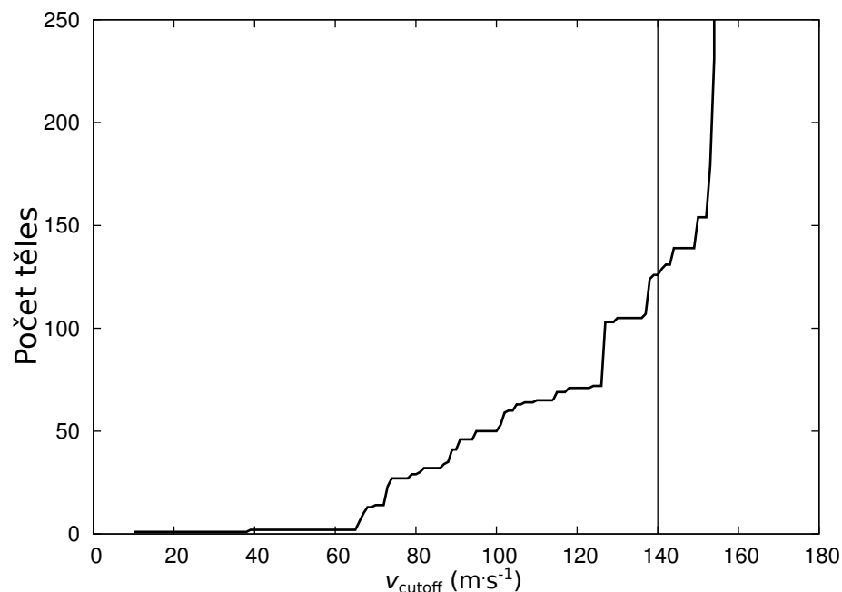
Obrázek 1.5: Příklad použití hierarchické shlukovací metody (HCM) — počet členů rodiny pro různé hodnoty v_{\text{cutoff}} pro rodinu Itha. Hodnota v_{\text{cutoff}} je vzdálenost tělesa v prostoru vlastních elementů od ostatních dosud identifikovaných těles. Od v_{\text{cutoff}} = 155 \text{ m}\cdot\text{s}^{-1} je zřetelný prudký nárůst počtu těles, tedy možné zahrnutí velkého množství těles z pozadí. Námí zvolená hodnota je v_{\text{cutoff}} = 140 \text{ m}\cdot\text{s}^{-1} .
