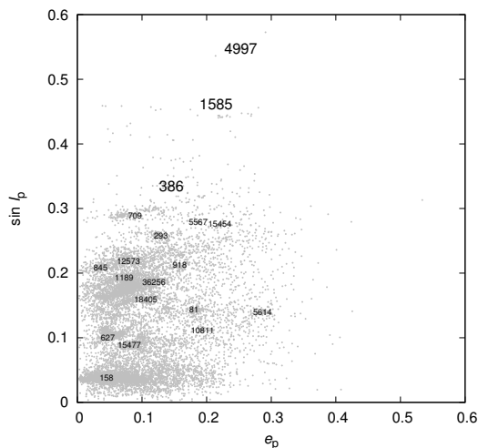
Obrázek 1.3: Obdoba obrázku 1.2, ovšem s větším rozsahem vlastních elementů. Kandidáti na nové rodiny objevení metodou „randombox“ jsou vyznačeny velkým číslem, dříve známé rodiny malým.
