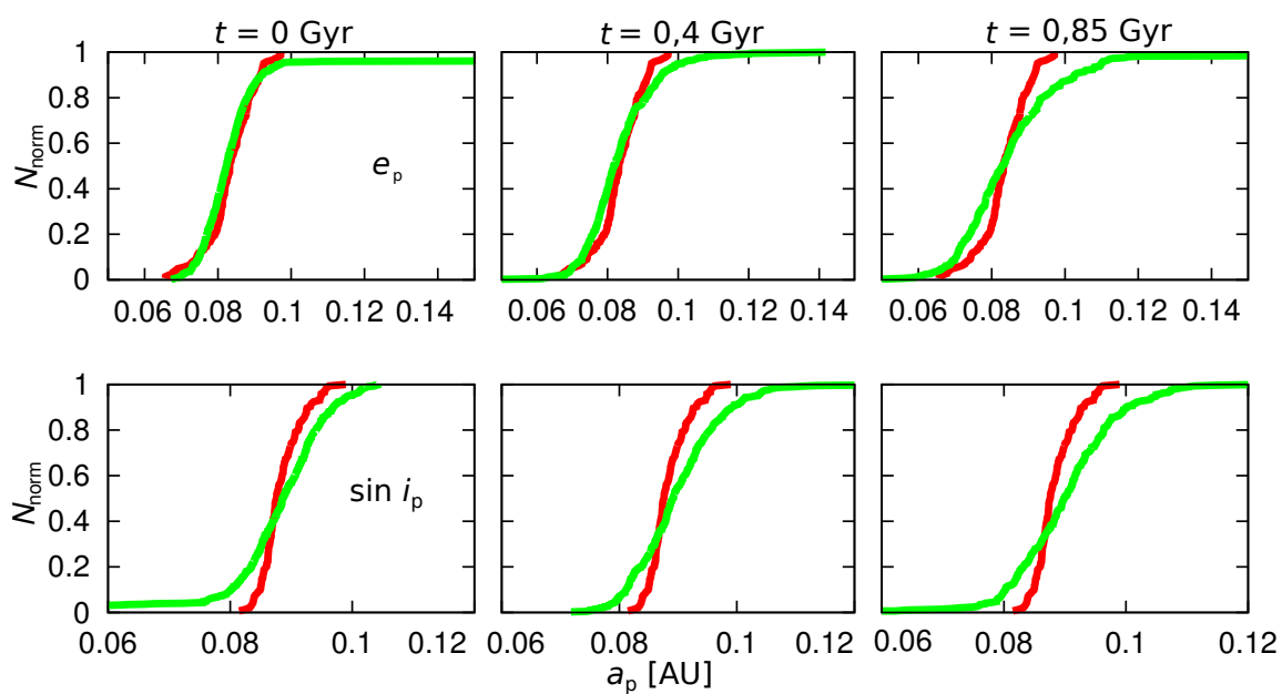
Obrázek 3.12: Normované kumulativní rozdělení vlastních excentricit a vlastních sklonů pozorovaných (červená) a simulovaných (zelená) těles rodiny 15477 během vývoje po dobu 0,85 Gyr. Pozorovaná tělesa jsou vybrána hierarchickou shlukovací metodou.
