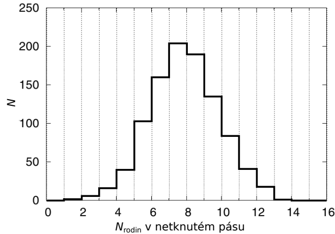
Obrázek 2: Histogram očekávaného počtu velkých rodin (s velikostí mateřského tělesa D_{\text{PB}} > 100 km) v „netknutém” pásu vzniklých při velkém pozdním bombardování (Brož et al. 2013). V práci byl použit model orbitální nestability obřích planet, která měla za následek přesun transneptunických těles do vnitřní části sluneční soustavy. Na základě předpokládaného rozdělení velikostí těchto projektilů a orbitálního vývoje planet a transneptunických těles dle Vokrouhlický et al. (2008) bylo kolizními modely zjišťováno, kolik rodin mohlo vzniknout srážkami s těmito projektily. Tento histogram vznikl tak, že se v modelu nechalo rozpadnout 100 náhodně vybraných těles hlavního pásu s průměrem D > 100 km a zjišťoval se výsledný počet rodin vzniklých v „netknutém” pásu. Toto se opakovalo 1000 krát. Cílem bylo odhadnout maximální počet rozpadů během velkého pozdního bombardování. Je vidět, že nejčastěji v „netknutém” pásu vzniklo osm takovýchto rodin, přičemž pravděpodobnost vzniku jen jediné je < 0,001 .
