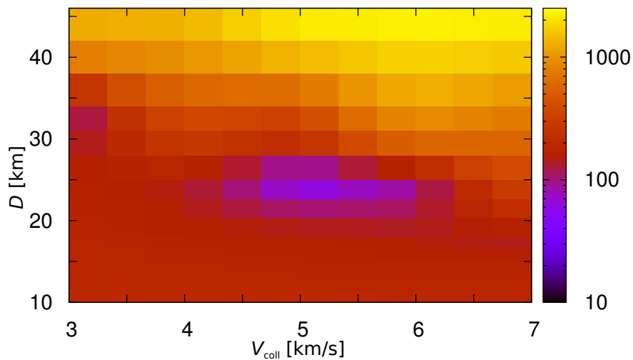
Obrázek 2.12: Závislost pseudo -\chi^2 (rovnice 2.2) pro srovnání syntetických rozdělení velikostí (Durda et al., 2007) a pozorované rodiny Itha na rychlosti srážky v_{\text{coll}} a velikosti projektilu D . Úhel srážky je ponechán konstantní, i_{\text{coll}} = 30^\circ .
