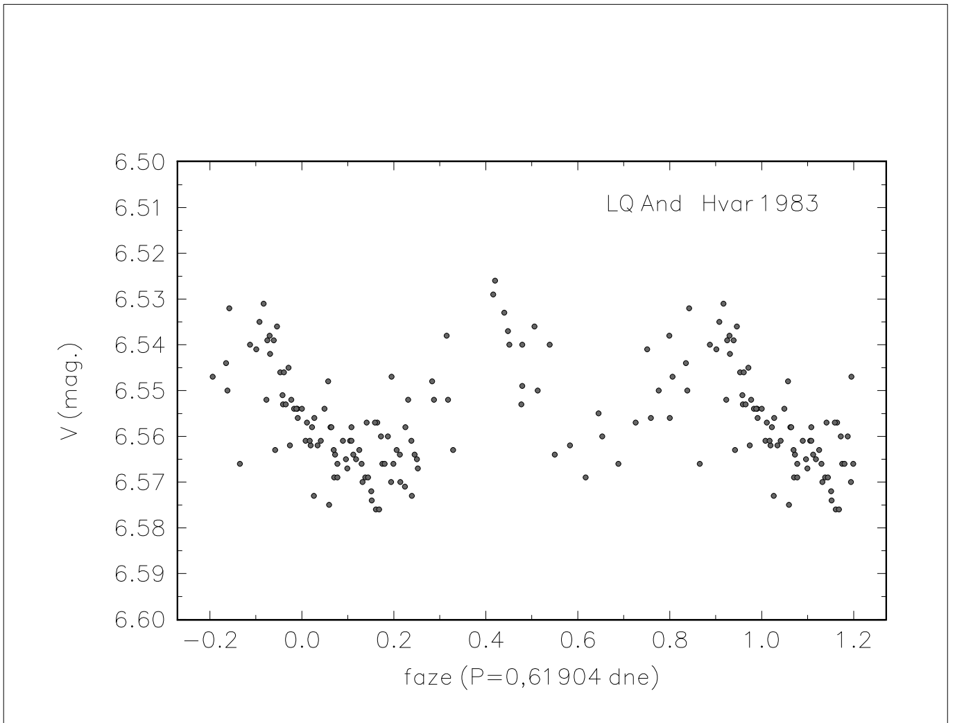
Obrázek 6: Světelná křivka LQ And pro data znázorněná na obr. 3 a pro nejlepší nalezenou periodu 0^d,61904 .
