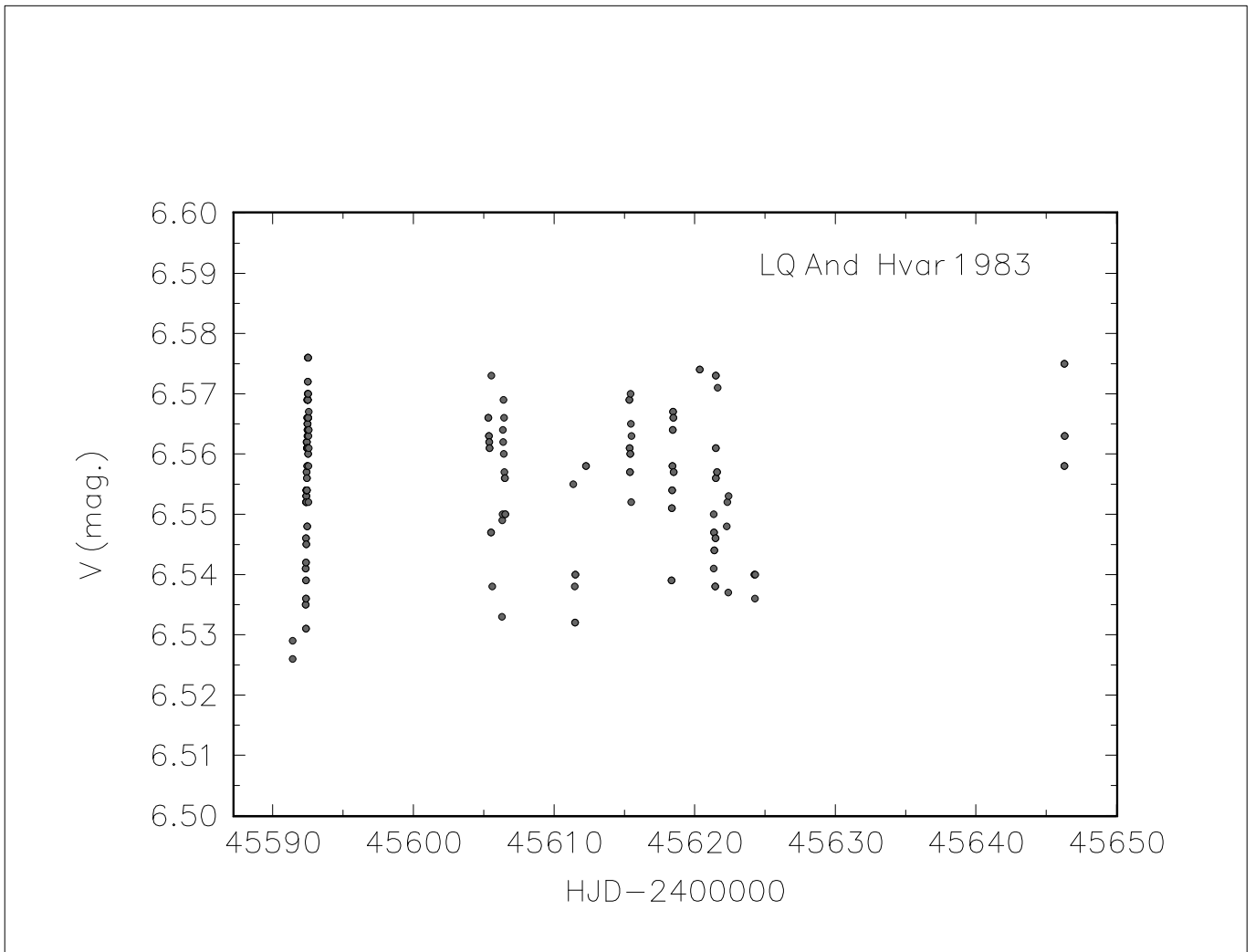
Obrázek 3: Změny jasnosti hvězdy se závojem LQ And, jak byly v Johnsonově filtru V naměřeny v sezóně 1983 na observatoři na Hvaru.
