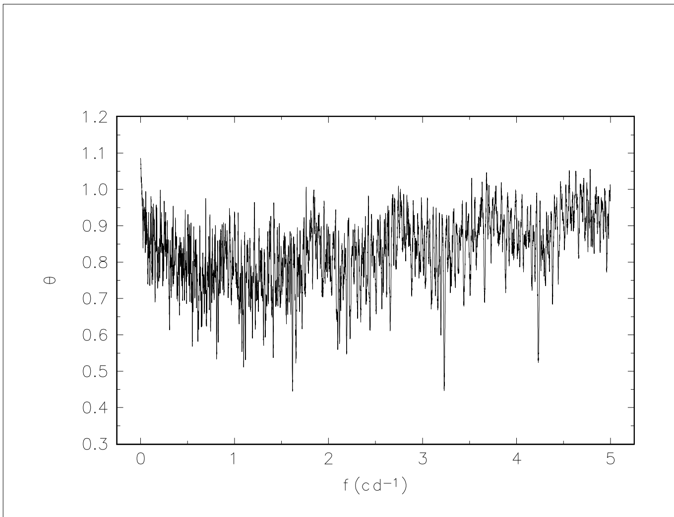
Obrázek 5: Ilustrace použití Stellingwerfovy metody na data LQ And znázorněná na obr. 3: V tomto periodogramu odpovídají nejlepší nalezené periody minimům \vartheta statistiky.
