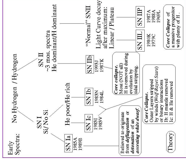
Obr. 7 — Klasifikační schéma supernov, rozvržené se zvýšeným zřetelem na jejich spektrální vlastnosti. V levé části diagramu jsou supernovy, jež nevykazují ve spektrech přítomnost vodíku (typ I, zahrnující podtypy Ia, Ib a Ic), v pravé části pak supernovy, u nichž bývá ve spektrech tento prvek detekován (typ II, s podtypy IIL, IIP a přechodovým podtypem IIb). Vzácná podtřída IIn na diagramu chybí. Převzato z ( http://www.astro.uu.nl/~langer/f3/transients/snobs.html ).
