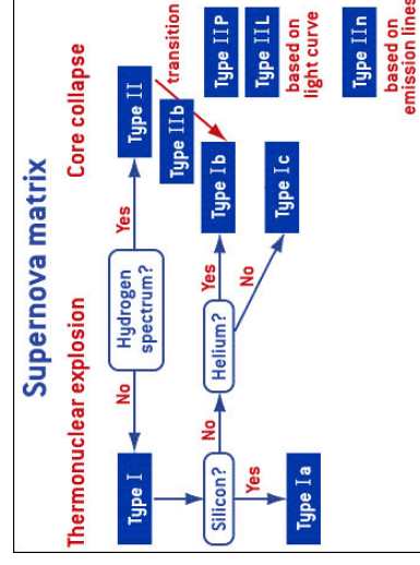
Obr. 8 — Klasifikační schéma supernov, uspořádané se zdůrazněním způsobu jejich vzniku. V levé části diagramu se nalézá osamocené typ Ia, vznikající termonukleární explozí bílého trpaslíka, v pravé části jsou nahlučeny supernovy, jejichž původ je v gravitačním zhroucení jádra jejich hmotného progenitora: typ II (s podtypy IIP, IIL, IIb a IIn) a dále typy Ib a Ic. Převzato z ( http://www.astronomy.com/en/Web%20Extras/2004/08/Know%20your%20supernovae.aspx ).
