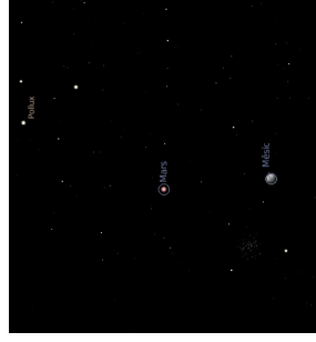
Obr. 20 — Konjunkce Marsu a Měsíce 25. 3., kvazikonjunkce Venuše a Merkuru 4. 4. a přiblížení Marsu k Jesličkám 17. 4. Mapky byly vytvořeny programem Stellarium.
