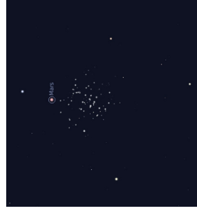
Obr. 20 — Konjunkce Marsu a Měsíce 25. 3., kvazikonjunkce Venuše a Merkuru 4. 4. a přiblížení Marsu k Jesličkám 17. 4. Mapky byly vytvořeny programem Stellarium.
