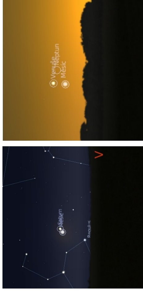
Obr. 7 — (a) Konjunkce Saturnu s Měsícem 10. 12.; (b) seskupení Jupitera, Marsu a Merkuru 11. 12.; (c) konjunkce Saturnu a Měsíce 6. 1.; (d) konjunkce Venuše a Měsíce 20. 1.
