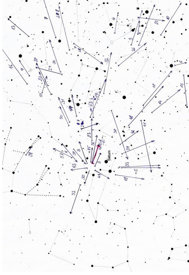
Obr. 5 — Pozorované meteory vynesené do gnomonické mapy.
