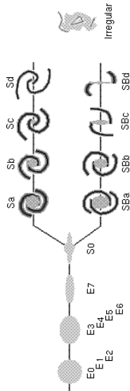
Obr. 1 — „Hubbleova ladička“ (rozšířená o spirální galaxie Sd a nepravidelné galaxie Irr) v níž je čočková galaxie znázorněna tak, jak vyhlíží při pohledu „zboku“. Převzato z [14].
