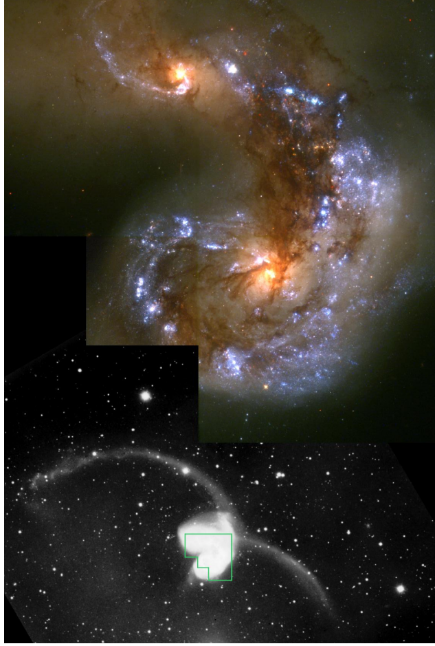
Obr. 19 — Dvojice NGC 4038/4039 Tykadla z Palomarské přehlídky a Hubblova dalekohledu. © Brad Whitmore (STScI) a NASA.
